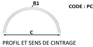
Main courante : Cintrage sens concave et convexe
