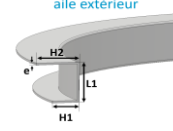
U : Cintrage convexe aile extérieur
