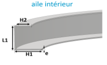
U : Cintrage convexe aile intérieur
