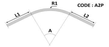
Arc avec deux partie droites
