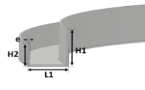
U : Cintrage sur chant 2
